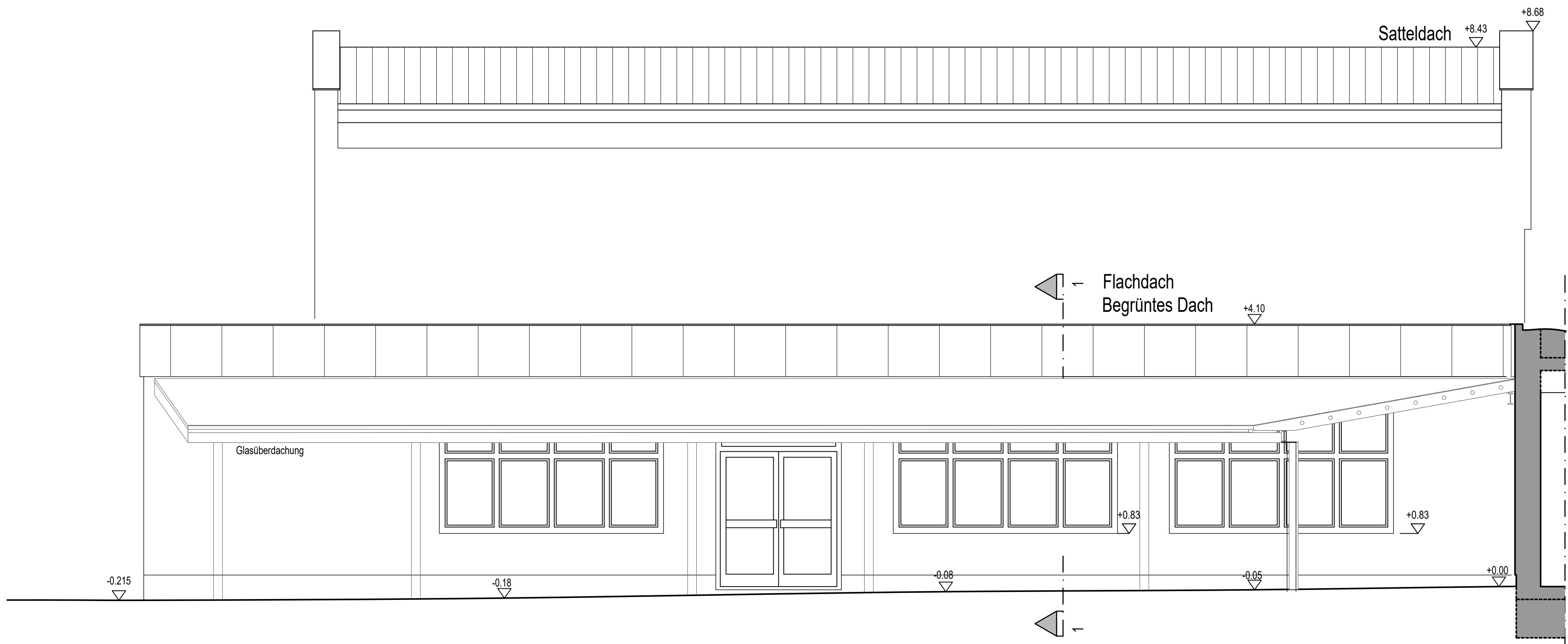
Ansicht West
